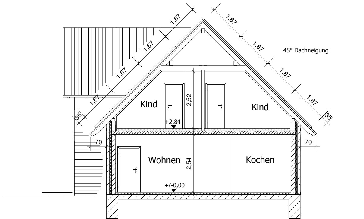
Schnitt A-A
