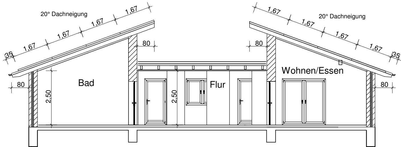
Schnitt A-A
