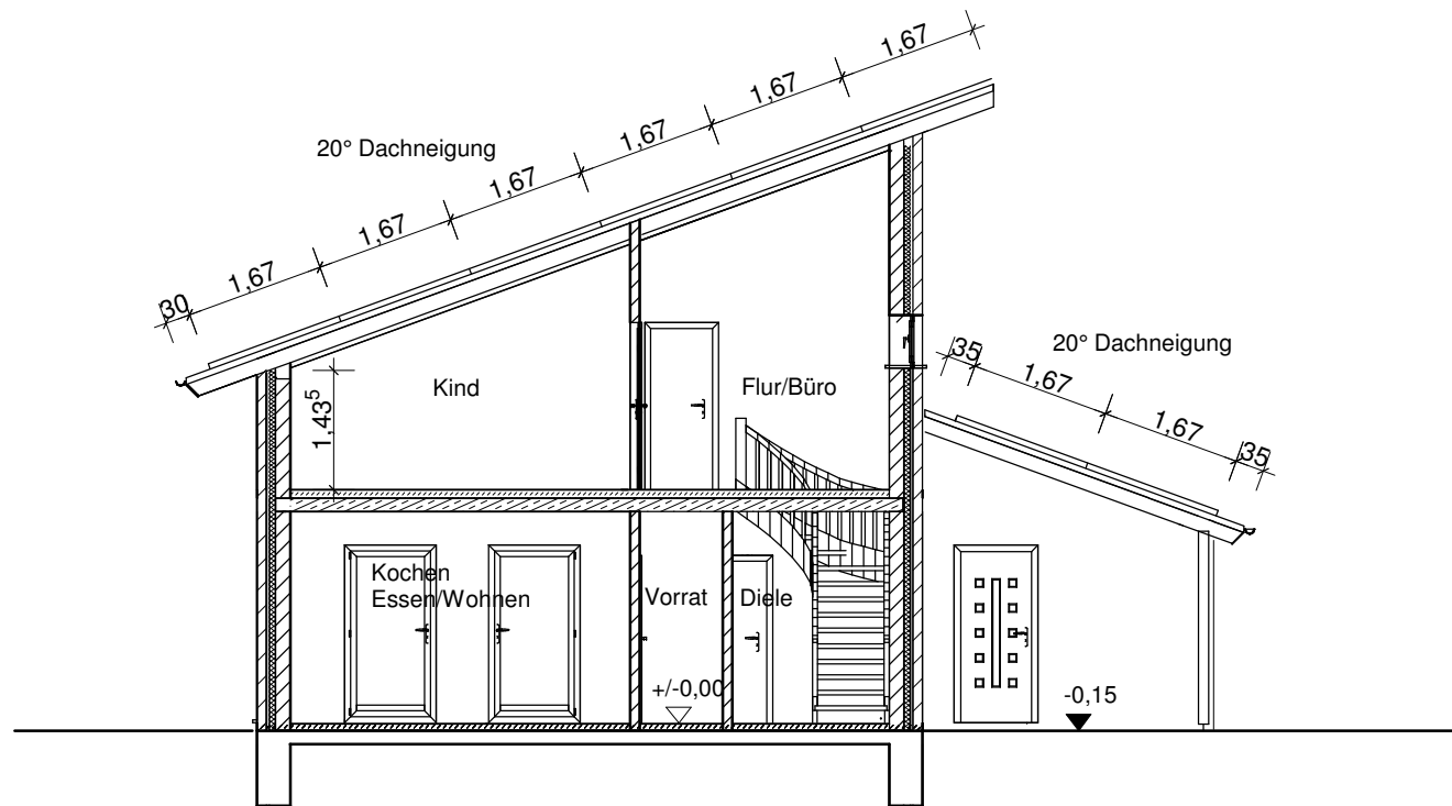
Schnitt A-A
