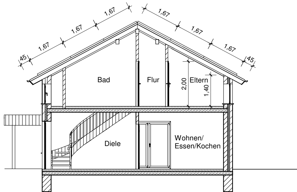
Schnitt A-A
