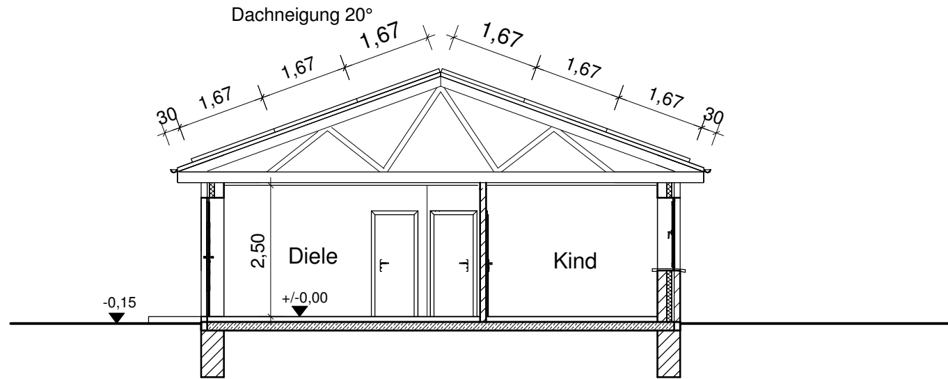
Schnitt A-A
