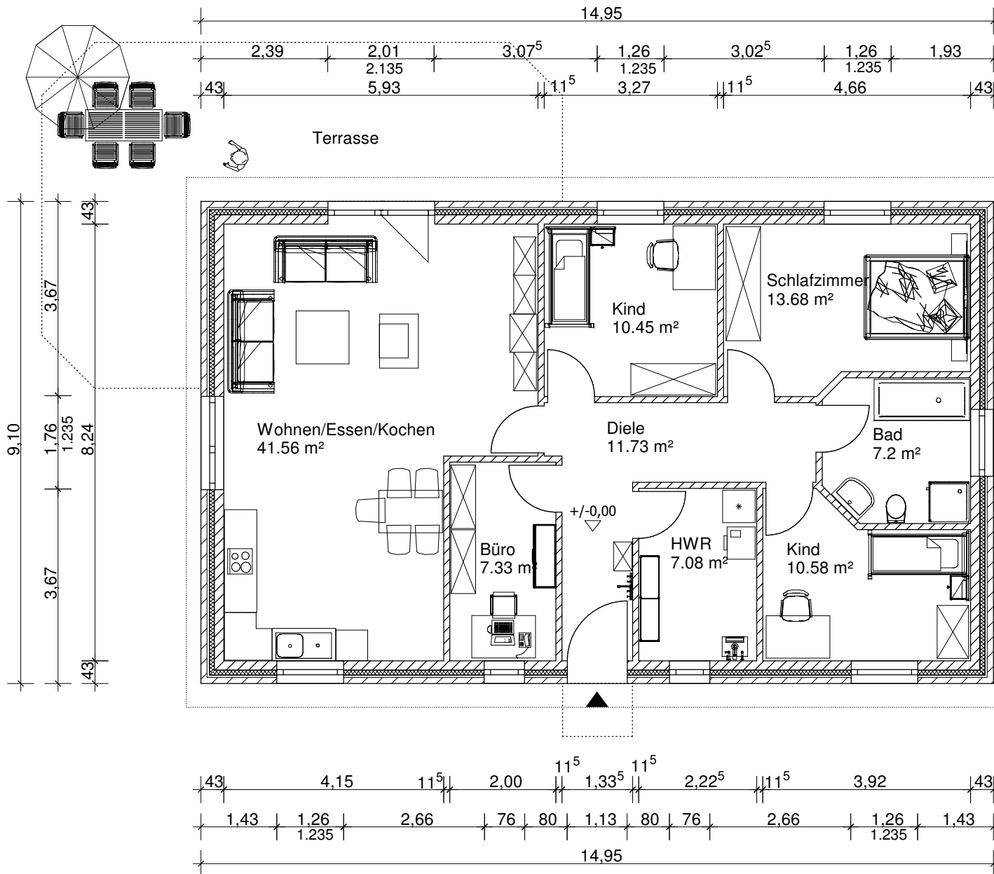
Grundriss-Erdgeschoss
